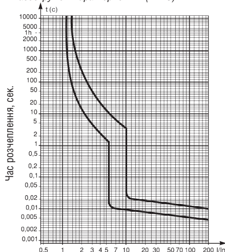
Часо-струмові характеристики (тип С)
