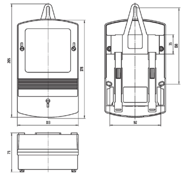
Габаритные и установочные размеры, мм
