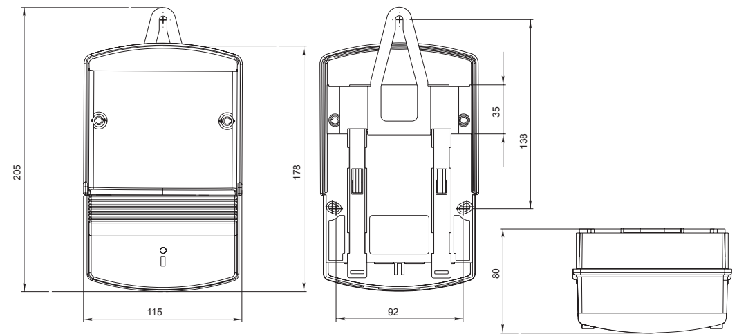
Габаритные и установочные размеры корпуса "В", мм
