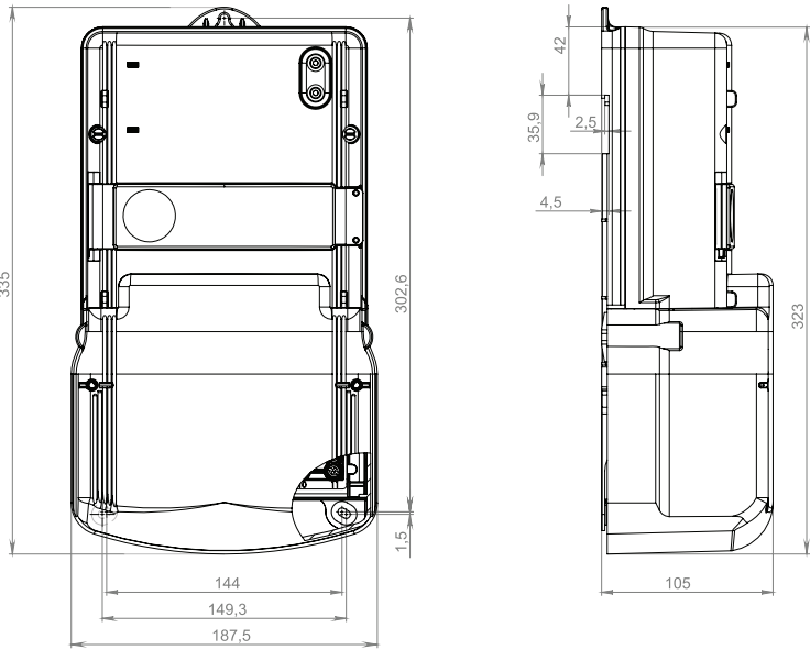
Габаритные и установочные размеры корпуса с реле до 120 А, мм
